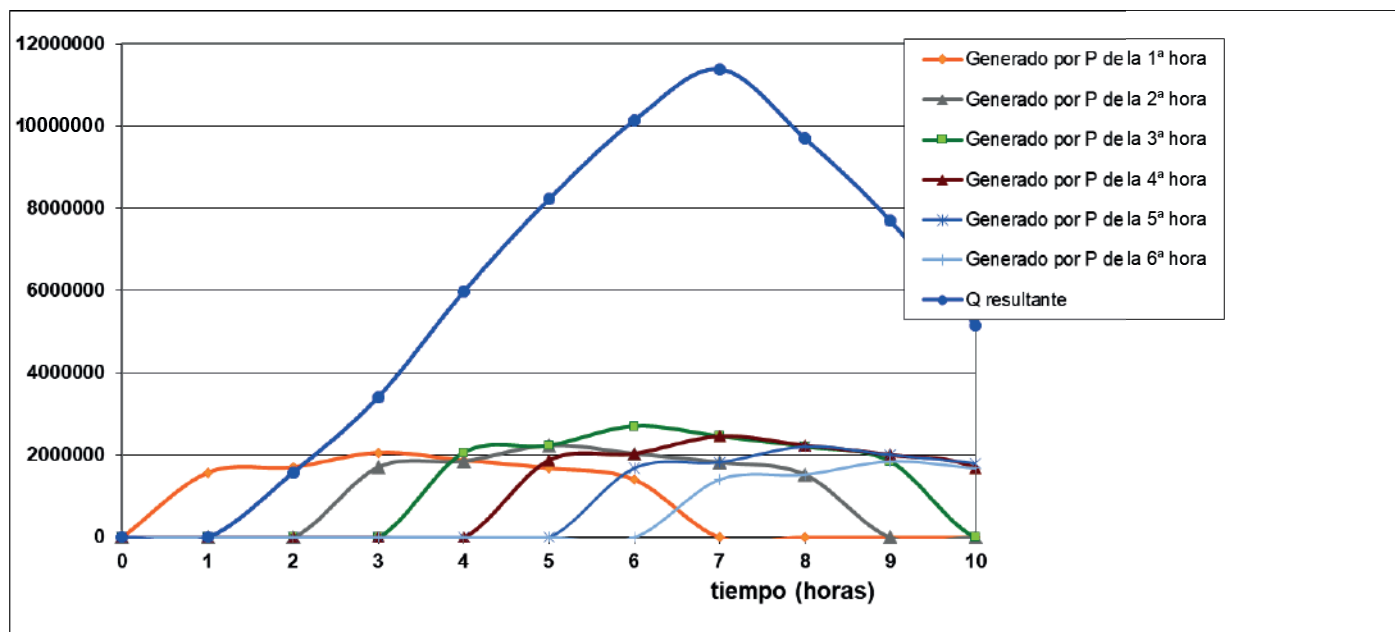
Gráfica 3. Hidrograma de la estación la Playa.
